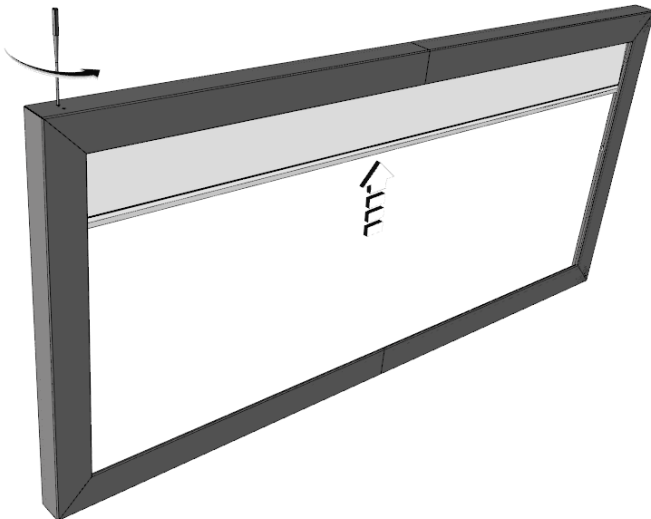
FORO VICINO AL MURO REGOLAZIONE FINE CORSA ALTO
